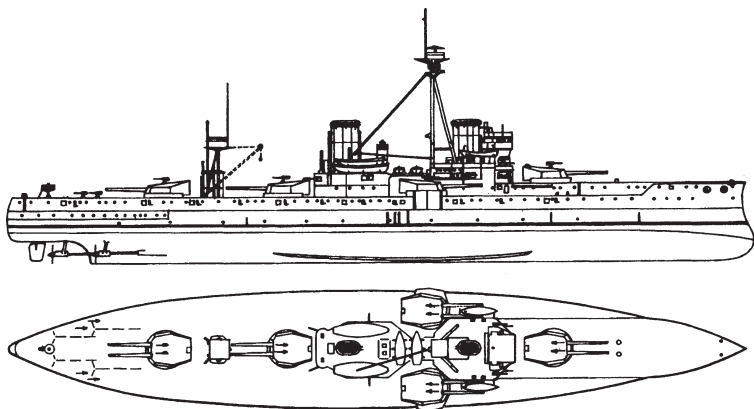
Линкор «Дредноут».
