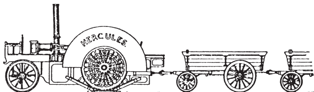
Безрельсовый локомотив, впервые примененный для военных нужд в 1854 году Д. Бовделем для перевозки грузов по самым тяжелым дорогам
