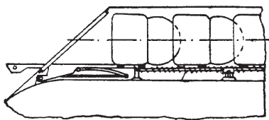
Схема устройства для постановки мин с подводного заградителя «Кrab»
